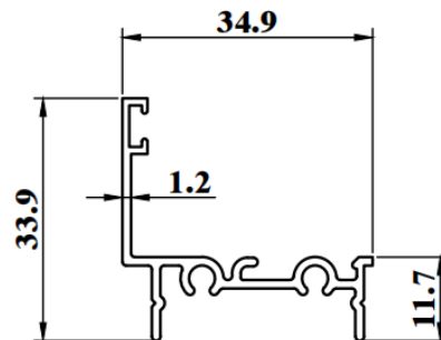
CW366G WEIGHT : 0.332 KG/M AP : 206.25mm
