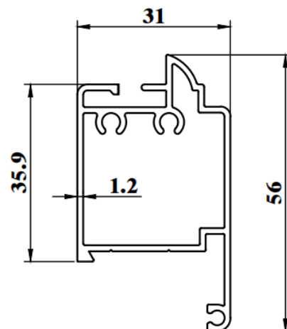
CW778G WEIGHT : 0.656 KG/M AP : 227.75mm
