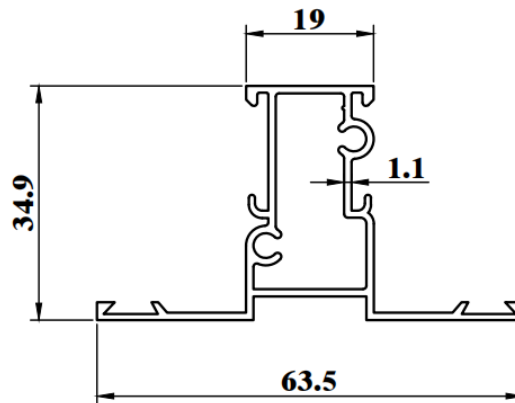
CW3711E WEIGHT : 0.551 KG/M AP : 260.10mm
